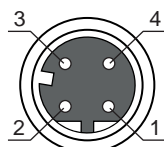
Figura 8.2: Assegnazione dei pin dell'interfaccia Ethernet
